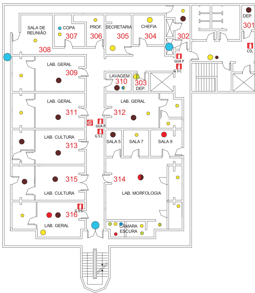
TERCEIRO PAVIMENTO
